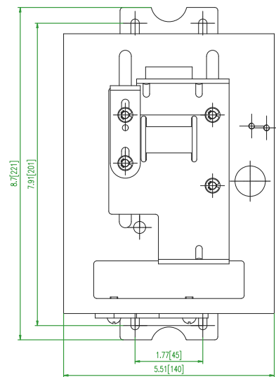
OMB23 Unit: in [mm]
